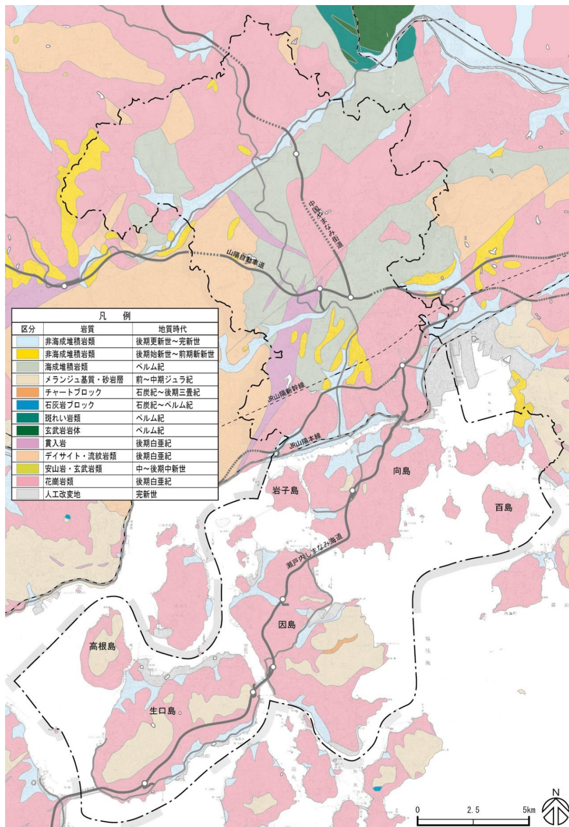
図 1-3 地質図
